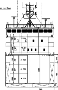
Bridgedeck
